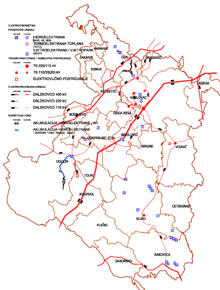
Kartogram XXIV: Energetski sustav – elektroenergetika; Izvor: PPKŽ, dokumentacija ŽPU KŽ
