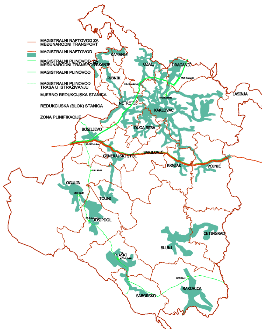
Kartogram XXVIII: Energetski sustav – proizvodnja i cijevni transport nafte i plina; Izvor: PPKŽ, dokumentacija ZPU KŽ;
